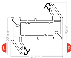
Transom Z EWS 7003
